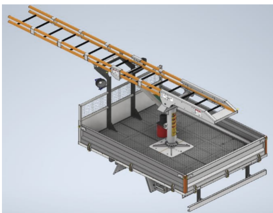
Figura 1 – Modelo de uma escada giratória central
