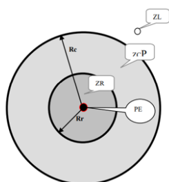
Figura 2 – ZR - zona de risco, ZC - zona controlada, ZL - zona livre, PE – ponto energizado (fonte: Ministério do Trabalho e Emprego, NR 10 – Segurança em Instalações e Serviços em Eletricidade, 2004, p. 15)
